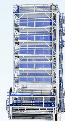
5層共押出フィルム生産設備
